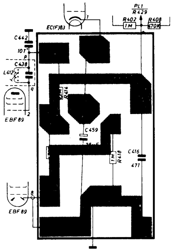
Bedruckte Platte PL 3 Printed Circuit board PL 3
