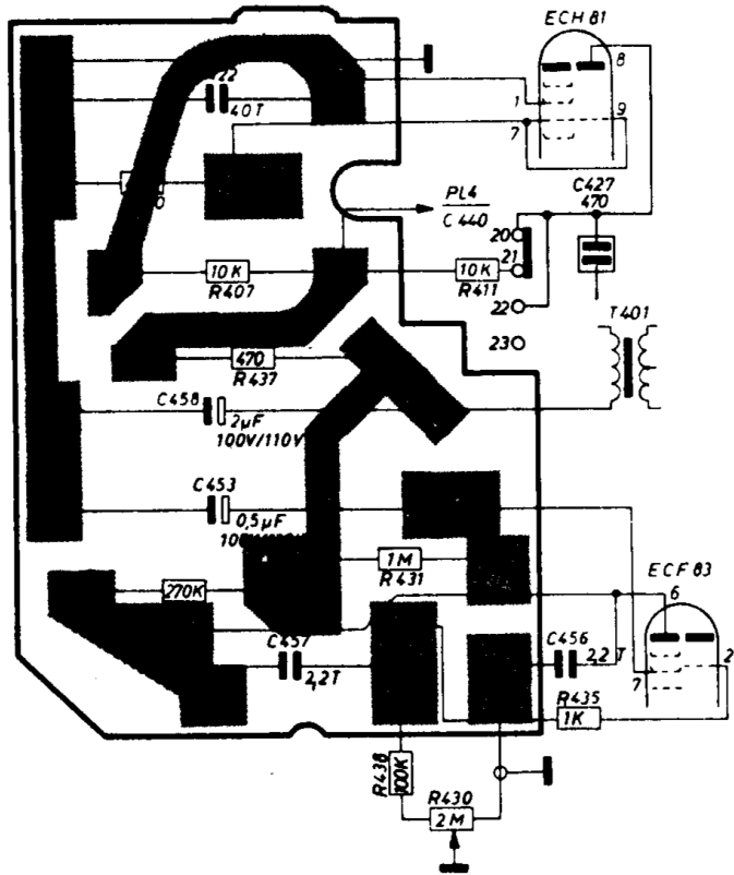
Bedruckte Platte PL 2 Printed Circuit board PL 2
